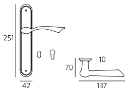
MAYPL05P MAYPL05Y Maniglia su placca Doorhandle on plate
