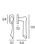
MAYDK01 Maniglia per finestra DK Windowhandle DK
