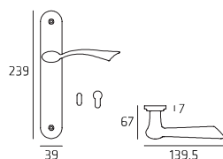
IDEPL04P IDEPL04Y Maniglia su placca Doorhandle on plate
