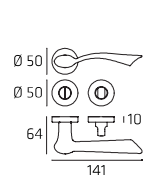
MAYR007W02 Maniglia per WC Doorhandle WC
